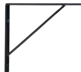
TE544 アイアン棚受け L 1,800円 (税込1,980円) サイズ/約w12 × d150 × h130mm 素材/鉄 ※木ネジ付 ※1本売りです
