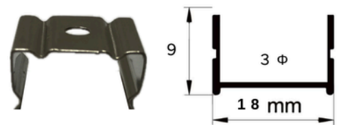
アルミプロファイル角型取付クリップ
