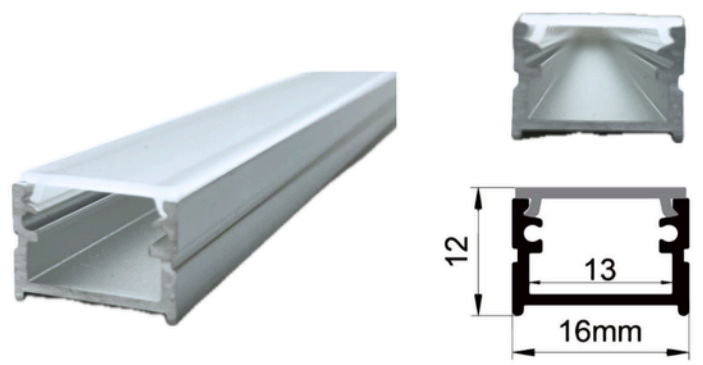
アルミプロファイル 角型
