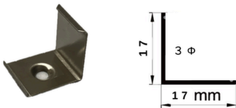
アルミプロファイル扇型取付クリップ
