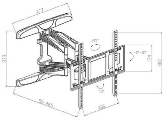
【寸法図 (mm)】
