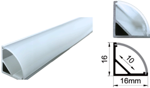
アルミプロファイル 扇形
